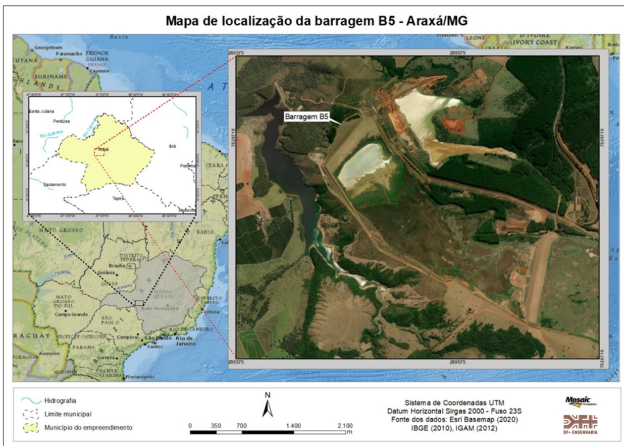
Figura 3.1 – Localização da Barragem B5.
