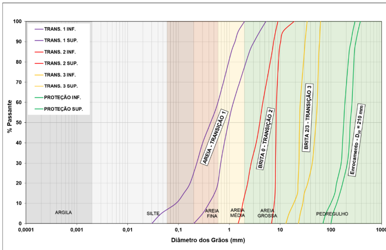
Figura 7.9 – Faixas granulométricas dos materiais granulares utilizados nas transições do canal periférico (29/01/2024).
