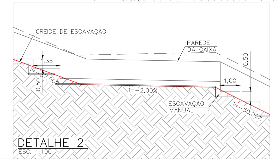
DETALHE 2 ESC. 1:100
