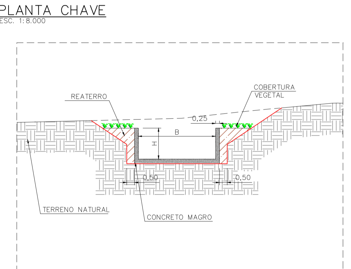
SEÇÃO TÍPICA RETANGULAR CPP-01 SEM ESCALA
